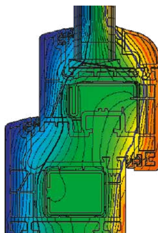
Tracé des isothermes Schüco Corona CT 70 Classic
