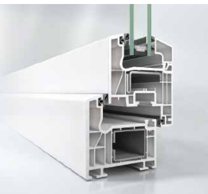
Schüco Corona CT 70 Classic
