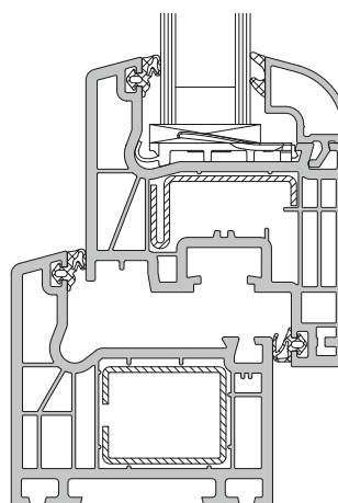
Schüco Corona CT 70 Classic Echelle 1:2
