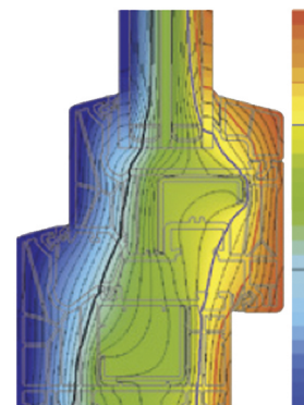
Isothermenverlauf Schüco Livng mit Mitteldichtung Isothermal flow in Schüco Livng with
